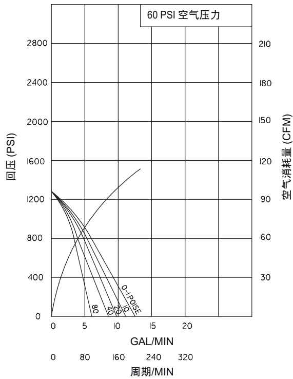
双球泵体, 6" 气动发动机, 6" 冲程, 23:1 比率
