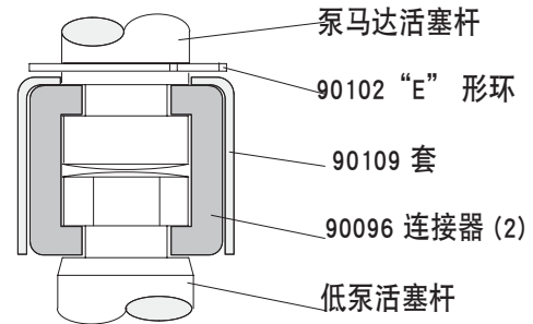
泵连接详图
